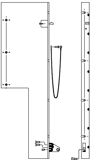
LEFT SIDE
