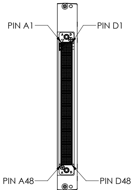
192 PIN RCV MODULE MATING FACE 510150115
