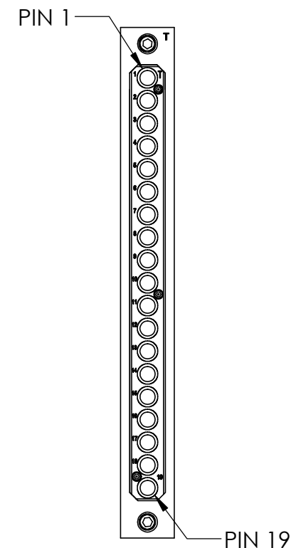
19 PN MCX RCV MATING FACE
