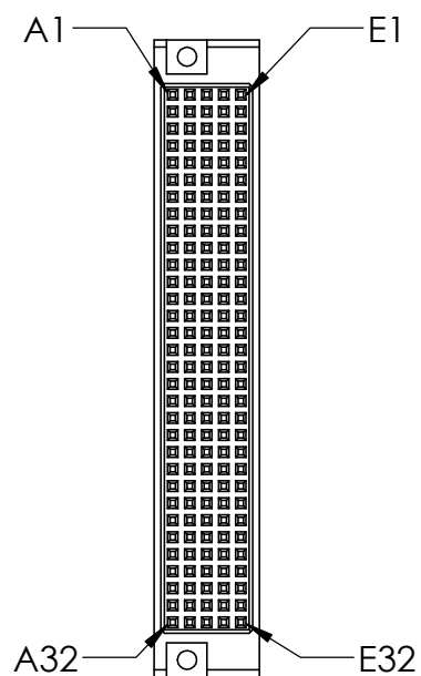
J1 MATING FACE 160 PIN FML DIN CONN
